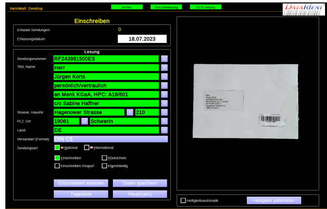
GUI-Beispiel
